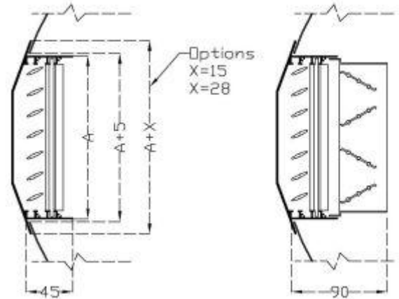
SK 2 עם שוליים מקופפים ורגיסטר RG
